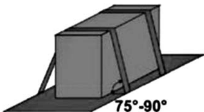
Rys. 6. Mocowanie odciążem przepasującym od góry
